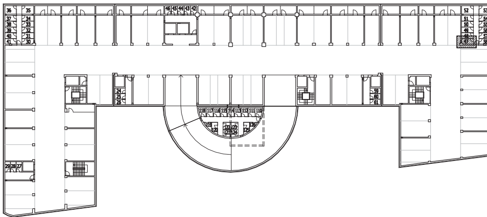
podrum -2
